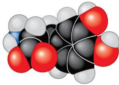
L-dopa
