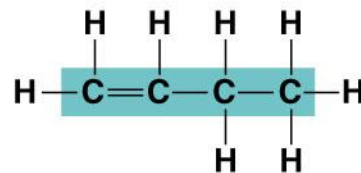
1-Butene
