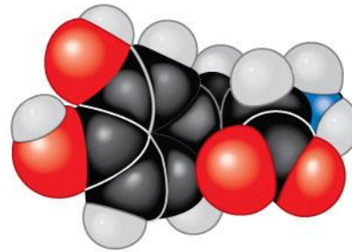
D-dopa
